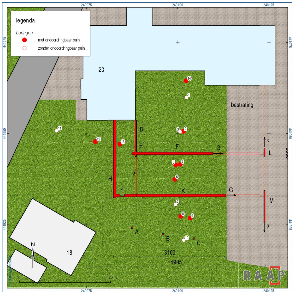
Figuur 5. Locatie van de tijdens werkzaamheden in de tuin in kaart gebrachte funderingen van het klooster (uit: De Graaf 2014) gecombineerd met de resultaten van het booronderzoek.
