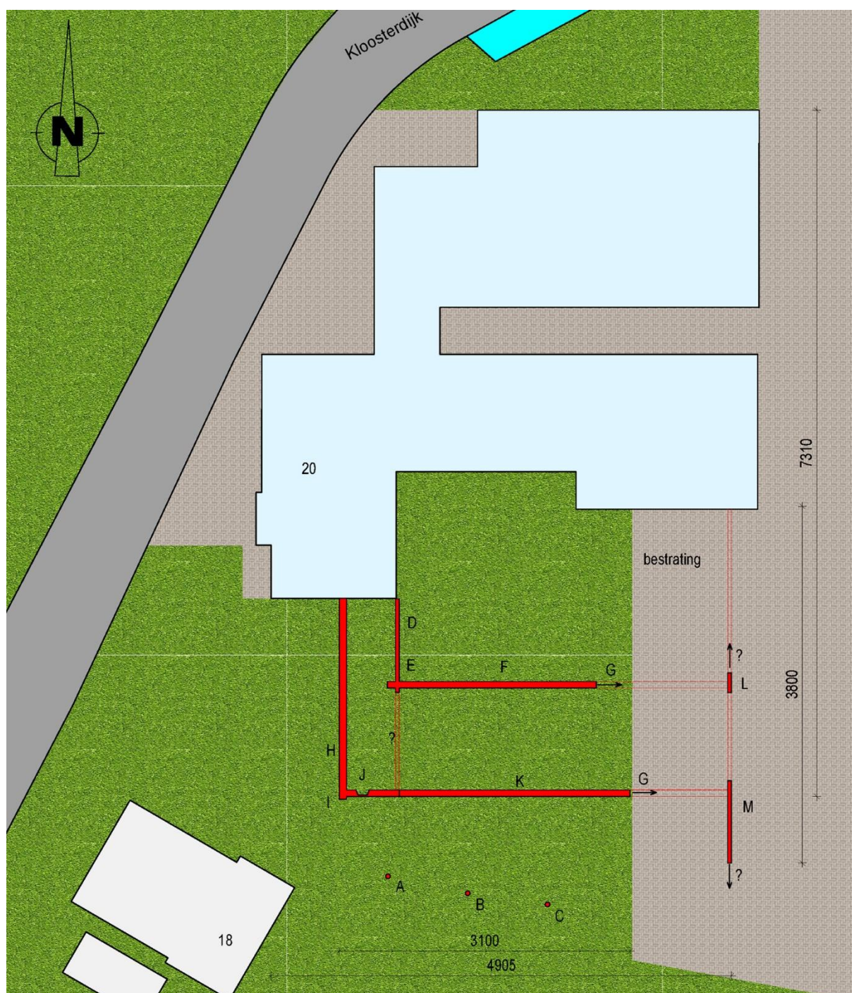
Figuur 3. Locatie van de tijdens werkzaamheden in de tuin in kaart gebrachte funderingen van het klooster (uit: De Graaf 2014).
