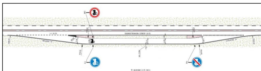
Gelderlandse standaard landbouwpasseerhavens (bron: Provincie Gelderland)
