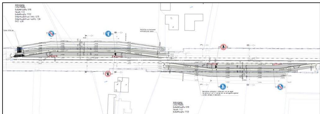
Weergave situatietekening deelloccatie 1 & 2 (bron: Provincie Gelderland)
